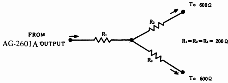
Fig. 2-2 Stereo input pad.
